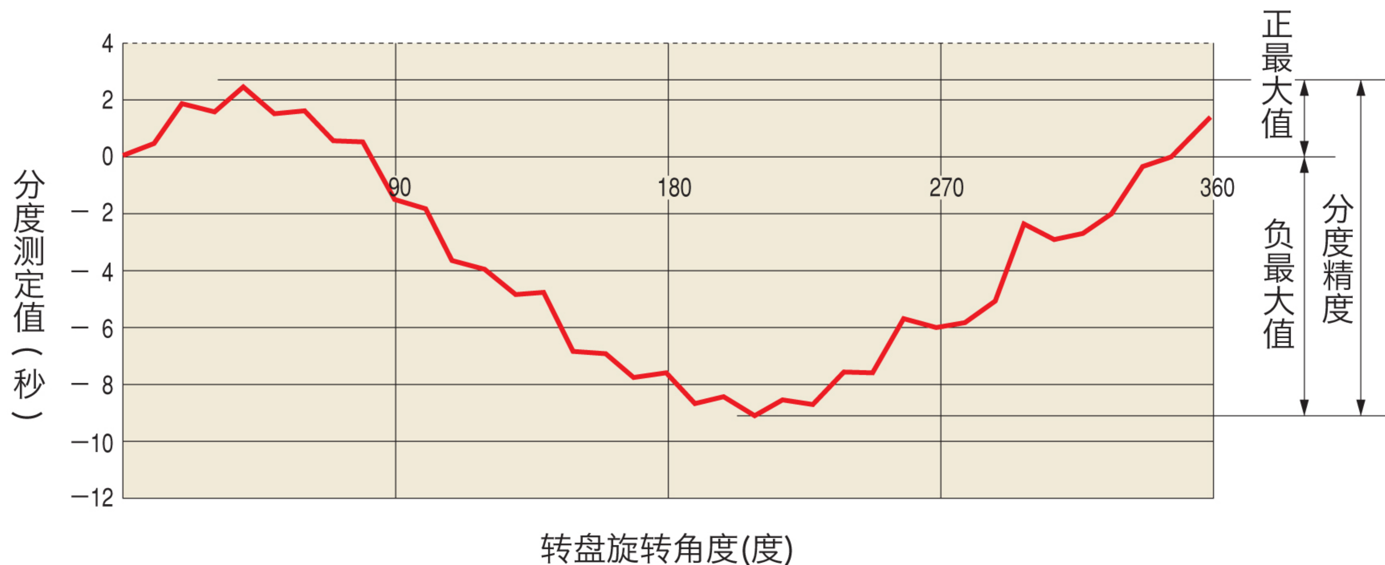
转盘的旋转角度及分度测定值
